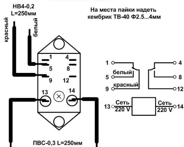
Модель реле: JZX-18FF 2CaAC220V2
