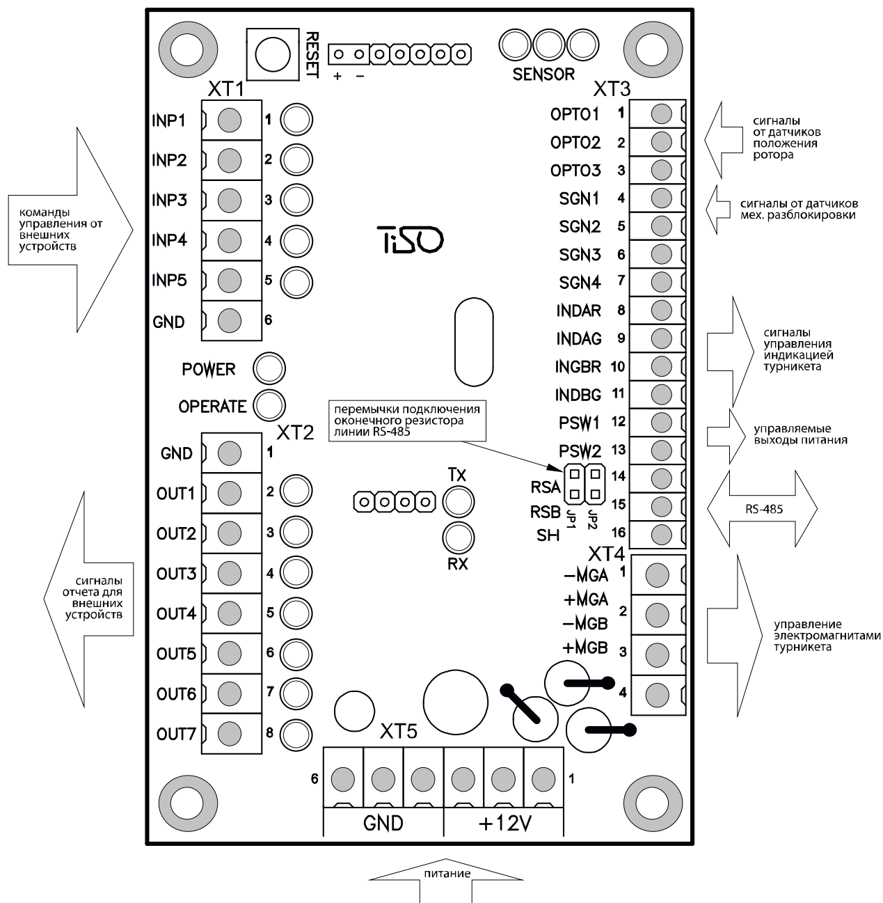
Рисунок 3 – Внешний вид контроллера PCB.112.21.20.00
